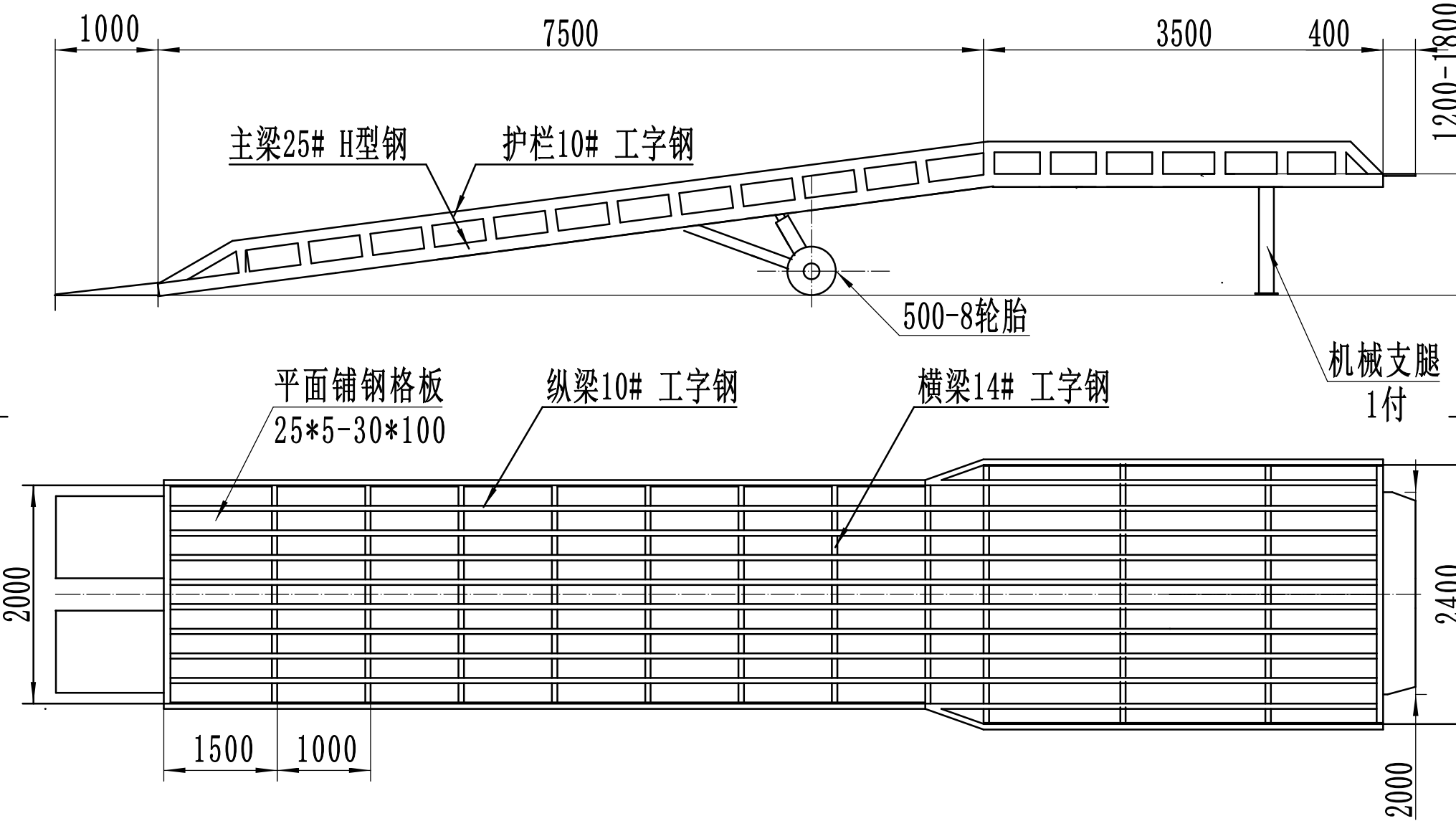
移动液压登车桥示意图
